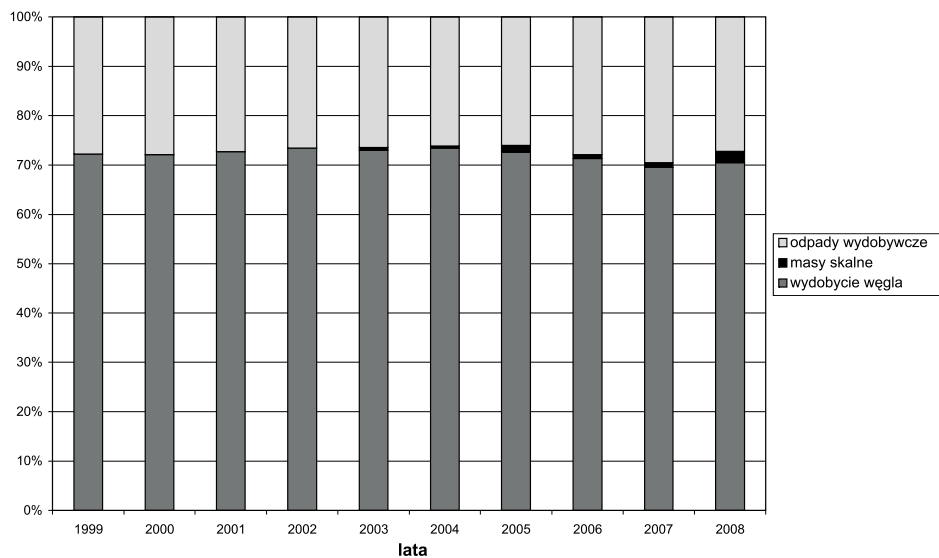
Rys. 3. Procentowy udział wydobytych ilości węgla i skały płonnej/odpadów wydobywczymi
