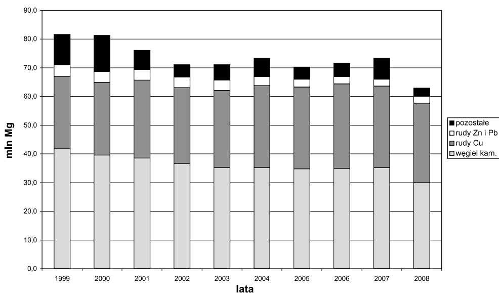
Rys. 1. Odpady wydobywcze według kopaliny
