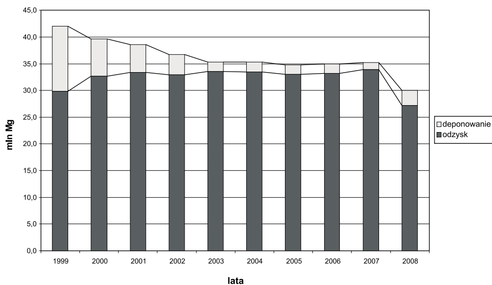
Rys. 2. Gospodarka odpadami wydobywczymi w górnictwie węgla kamiennego
