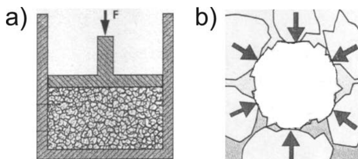
Rys. 4. Ściskanie kruszywa a) cylinder z kruszywem obciążanym stemplem prasy; b) ziarno ściskane w warstwie materiału
