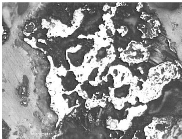
Fot. 5. Żużel po hutnictwie rud Zn-Pb; skupienia metaliczne; analiza mikroskopowa w świetle odbitym, 100×, 1N Phot. 5. Slag after Zn-Pb production; metallic aggregates; microscopic analysis in the reflected light, 100×, 1N
