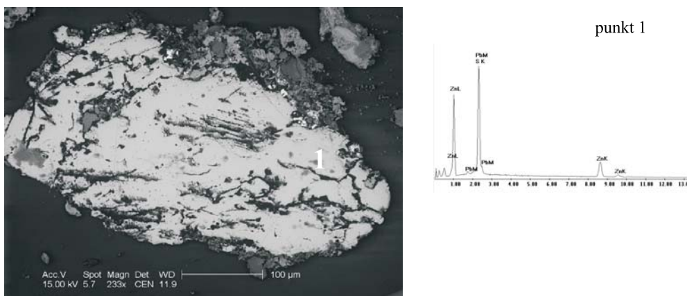
Fot. 4. Żużel po hutnictwie rud Zn-Pb; obraz z mikroskopii elektronowej wraz z interpretacją składu chemicznego; koncentracja ołowiu i cynku Phot. 4. Slag after Zn-Pb production; photo from electron microscopy with interpretation of the chemical composition; concentration of lead and zinc
