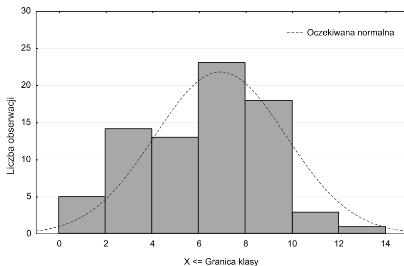
Rys. 6. Rozkład wartości porowatości utworów jury górnej-kredy dolnej
