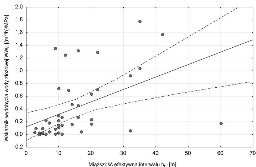
Rys. 9. Zależność wskaźnika wydobycia wody złożowej od miąższości efektywnej dla utworów jury górnej-kredy dolnej
