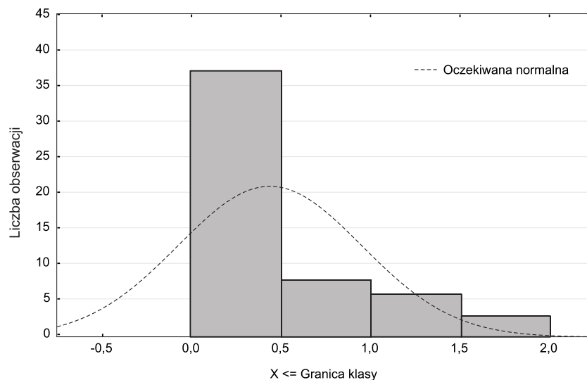
Rys. 3. Rozkład wartości wskaźnika wydajności wydobycia wody złożowej z utworów jury górnej-kredy dolnej
